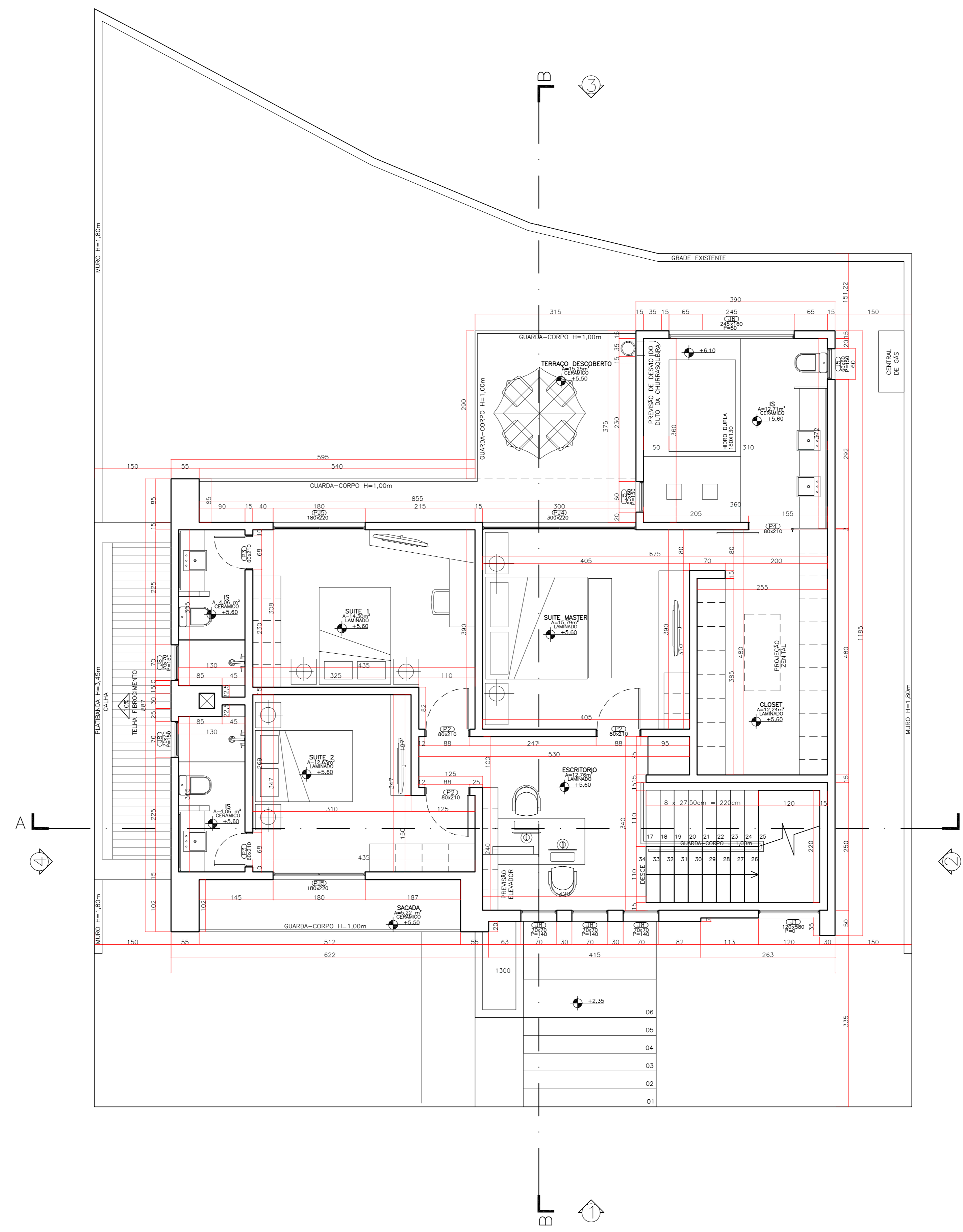
PLANTA SUPERIOR ESCALA 1/50
