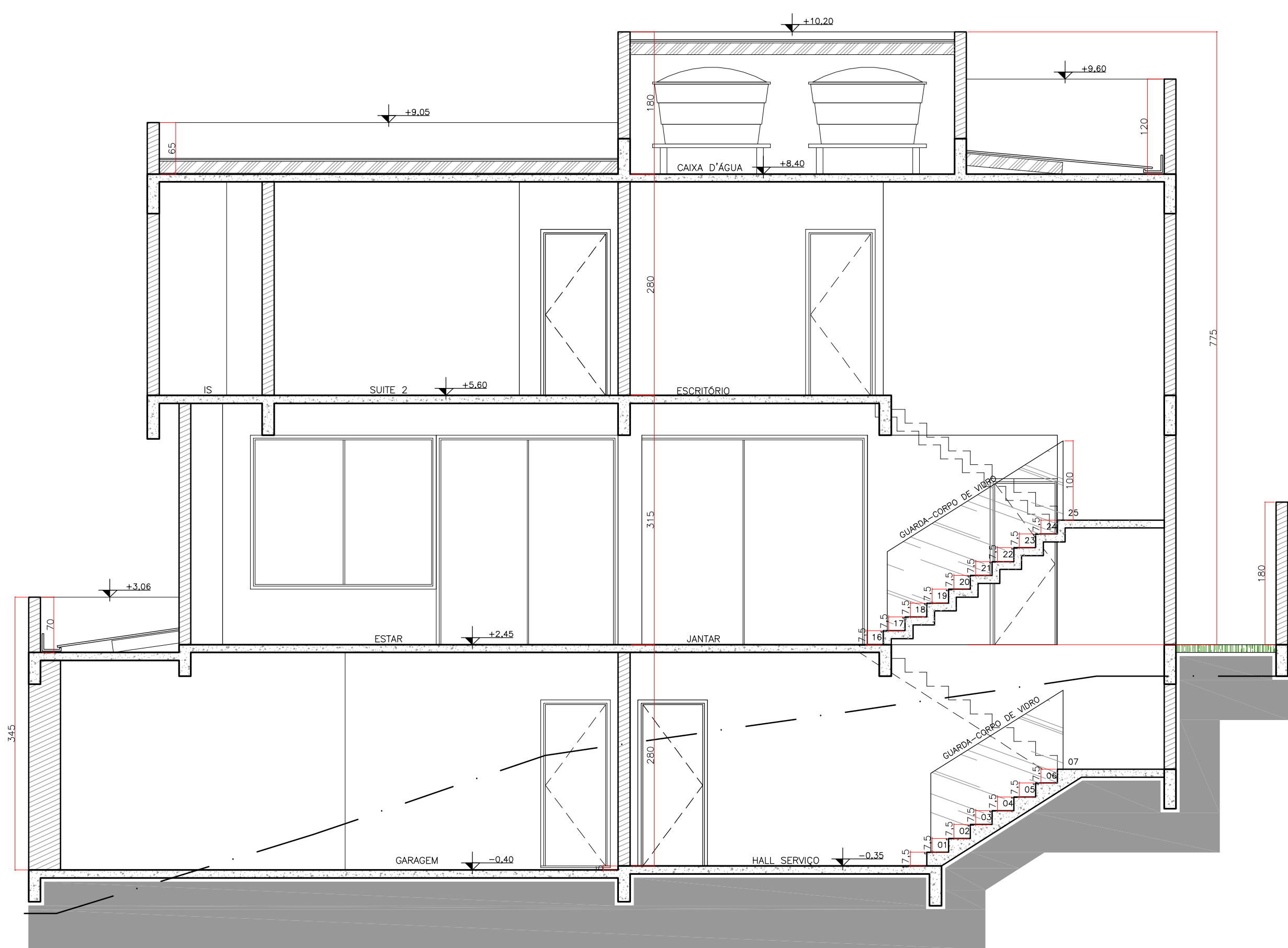
CORTE A ESCALA 1/50
